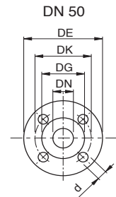
Flanges EN 1092-2 PN 25
